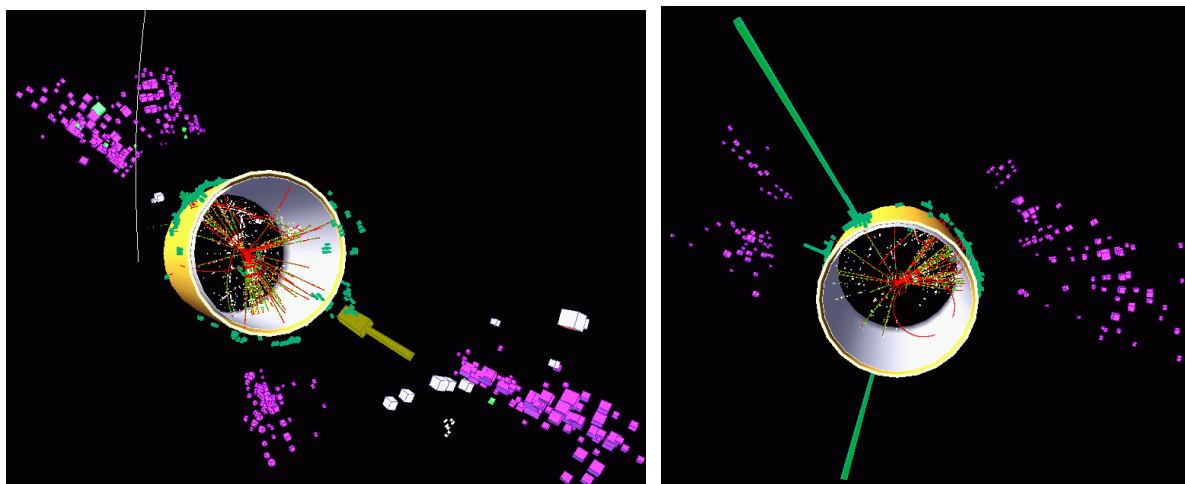
Obr.8) Případy, které by mohly být způsobeny rozpadem H a Z částic, pozorované experimentem OPAL. Vlevo rozpad ( H \rightarrow b\bar{b} ) ( Z \rightarrow q\bar{q} ) končící vytvořením čtyř výtrysků (čtyři široké hadronové spršky vyznačené fialovou barvou), vpravo případ ( H \rightarrow b\bar{b} ) ( Z \rightarrow l^+l^- ) končící dvěma hadronovými sprškami a dvěma úzkými elektromagnetickými sprškami (vyznačeny zelenou barvou). (Zdroje experimentu OPAL v CERNu)
