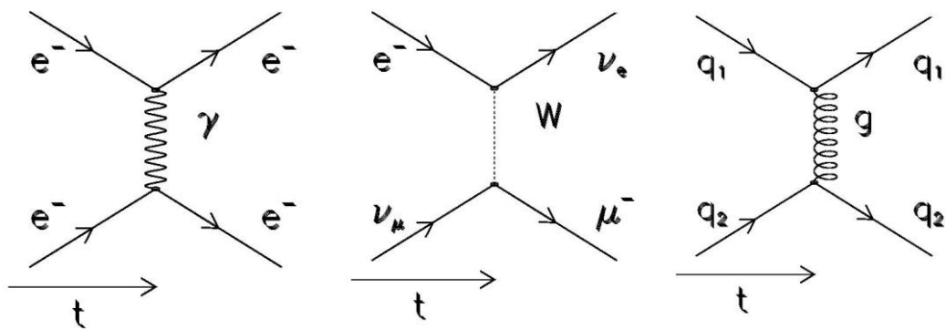
Obr.2) Výměnný charakter jednotlivých interakcí zobrazený pomocí Feynmanových diagramů. Příklady pro jednotlivé interakce: vlevo je elektromagnetická interakce - rozptyl dvojice elektronů zprostředkovaný virtuálním fotonem, uprostřed slabá interakce - reakce elektronu a mionového neutrína za vzniku mionu a elektronového neutrína zprostředkovaná virtuálním W bosonem a vpravo silná interakce - rozptyl kvarku na kvarku zprostředkovaný gluonem.
