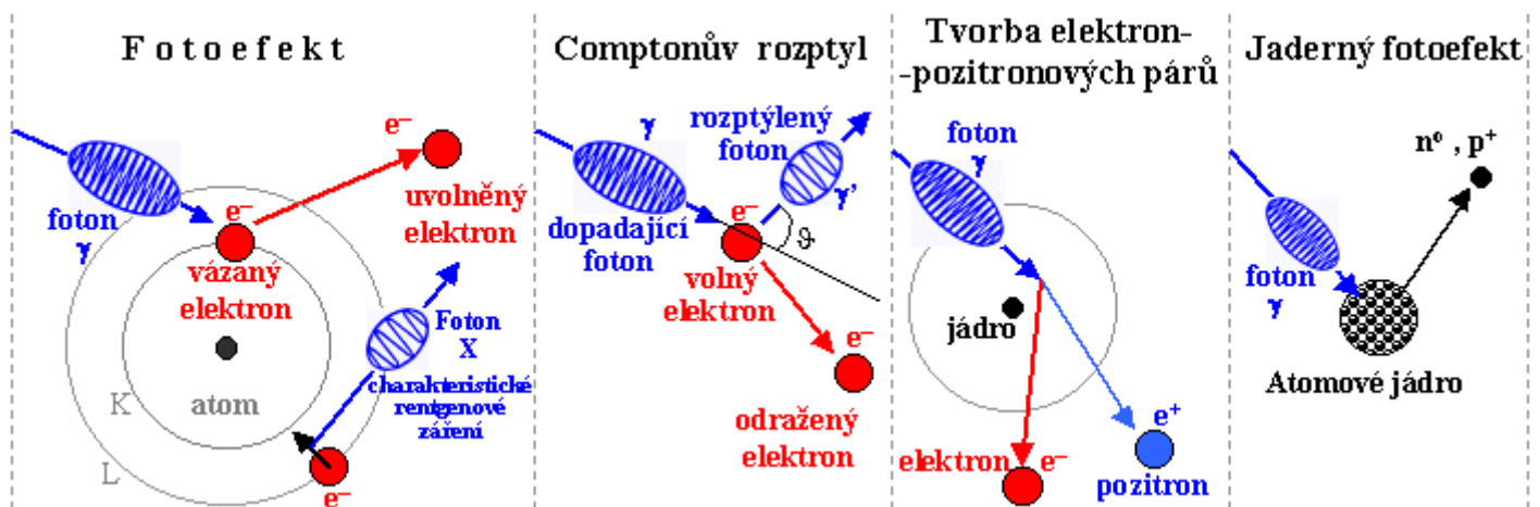
Obr.1.6.3. Čtyři způsoby interakce záření gama s látkou.
